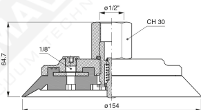
Art. AF 150 50
