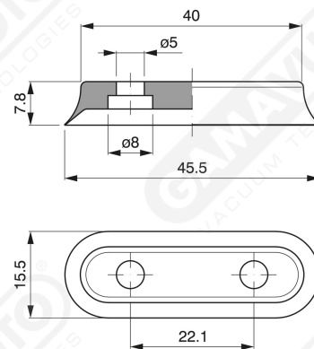
Art. VO 46
