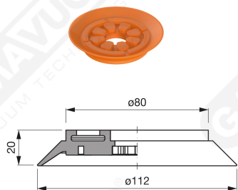
Art. VPF 110 45
