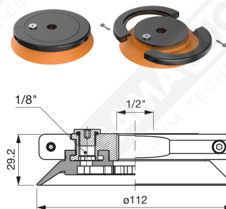
Art. VPF 110 63
